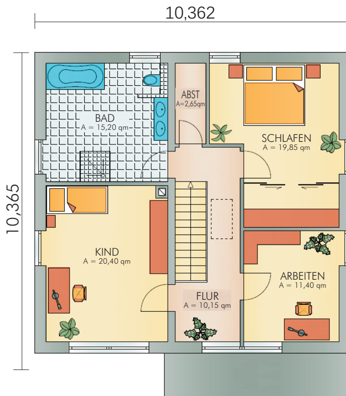
Obergeschoss
