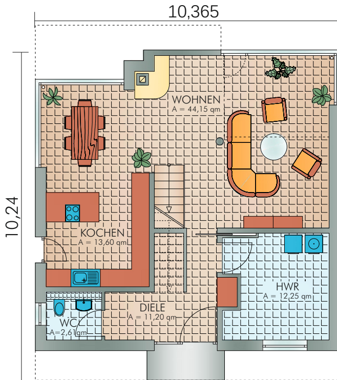
Erdgeschoss
